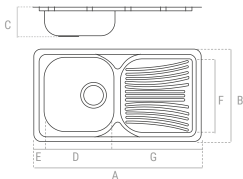
MEDIDAS FREGADERO | DIMENSIONS ÉVIER | SINK DIMENSIONS
