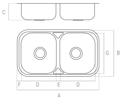
MEDIDAS FREGADERO | DIMENSIONS ÉVIER | SINK DIMENSIONS
